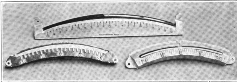
FIG. 15A. Liquid-Bubble Lateral Inclinometers
