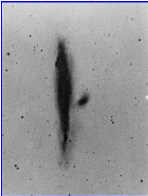
Arp 281
