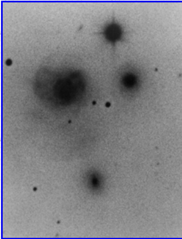
Arp 221
