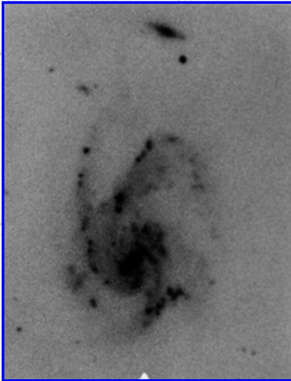
Arp 69
