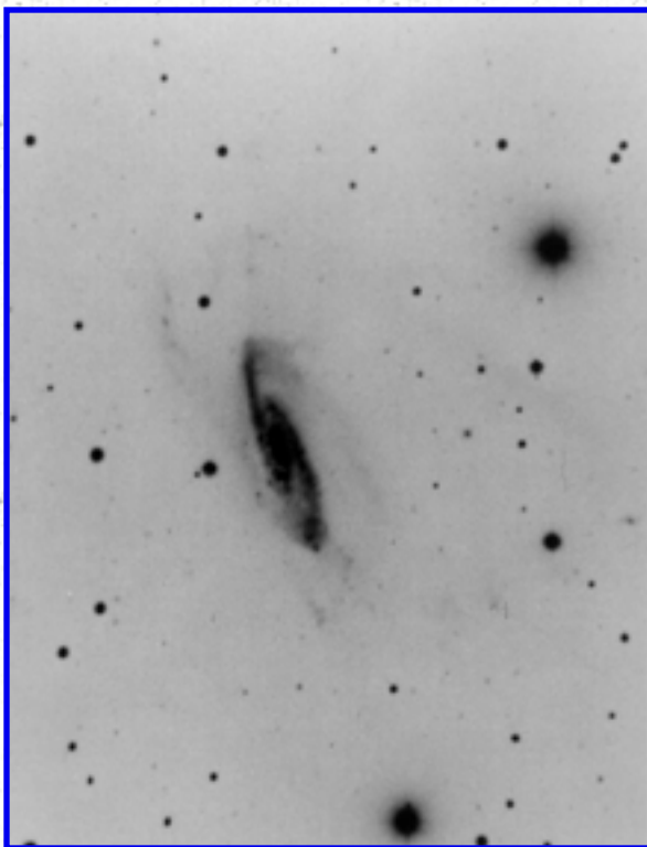
Arp 289
