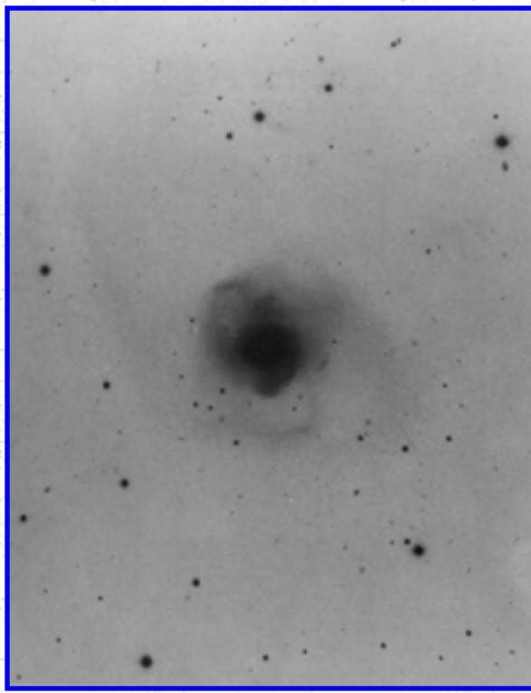
Arp 222
