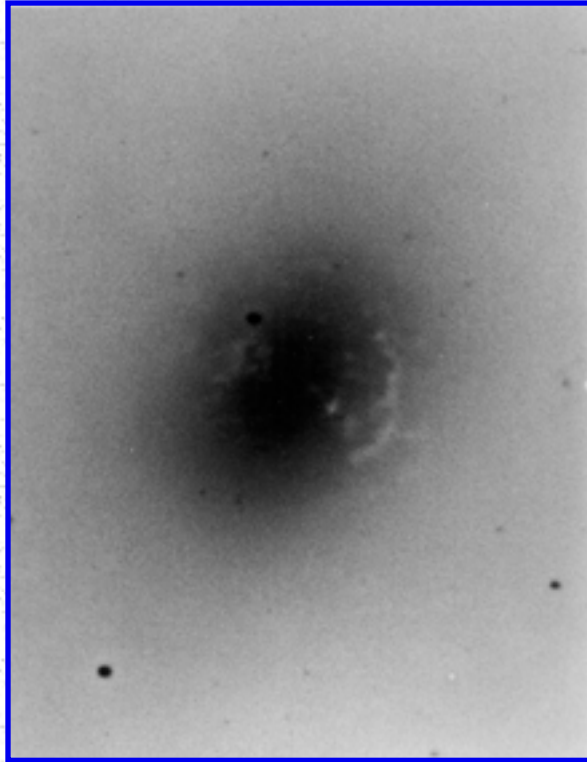
Arp 154
