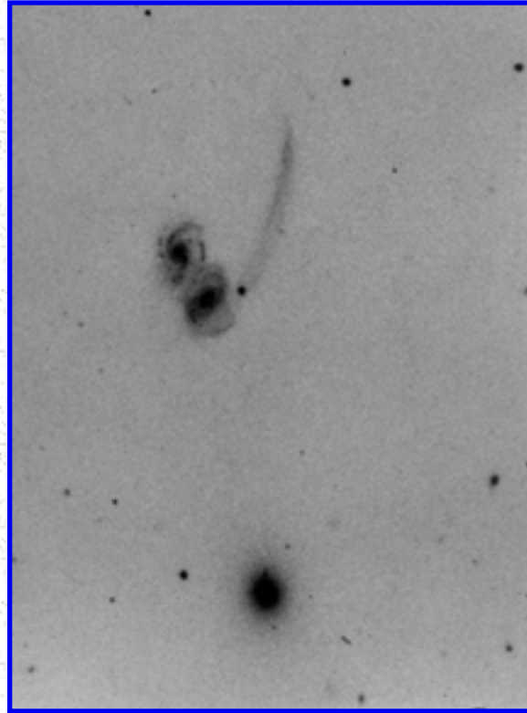
Arp 190
