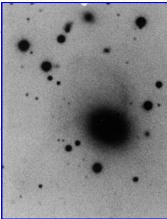
Arp 165
