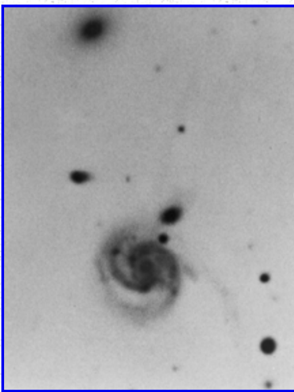
Arp 182
