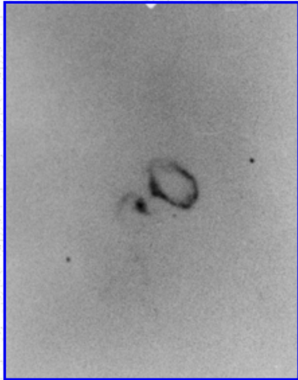
Arp 146
