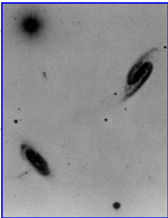
Arp 285
