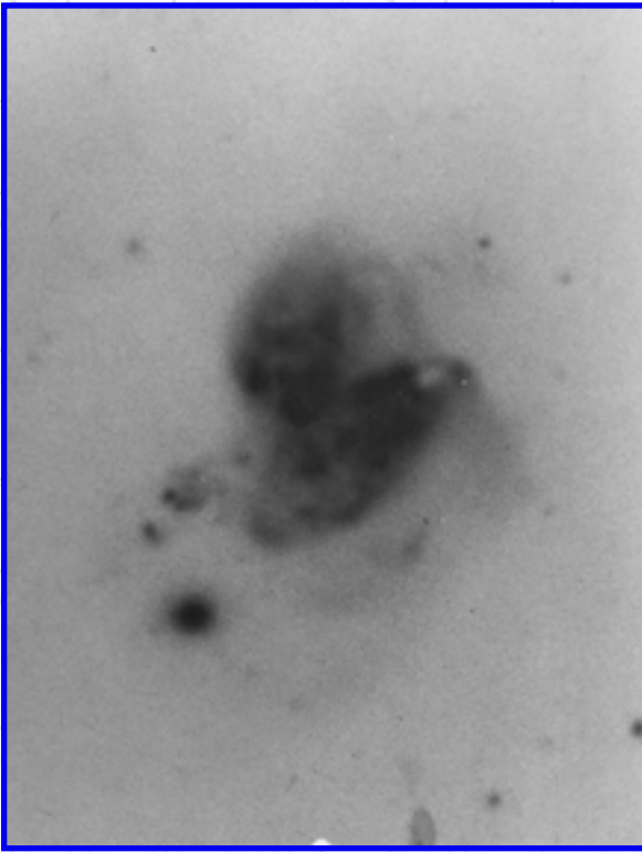
Arp 299
