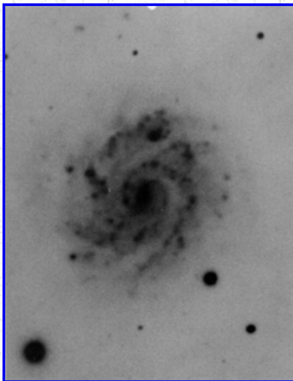
Arp 38
