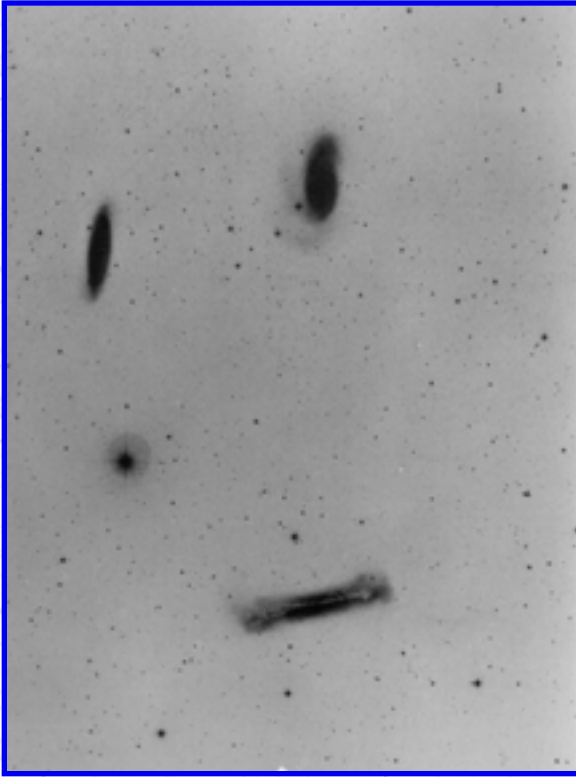
Arp 317
