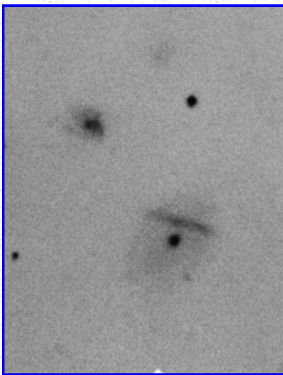
Arp 338
