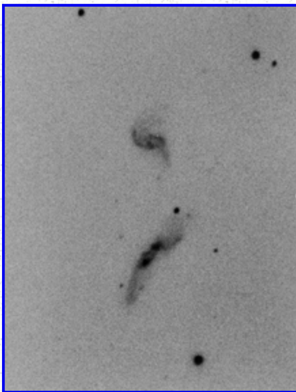
Arp 250
