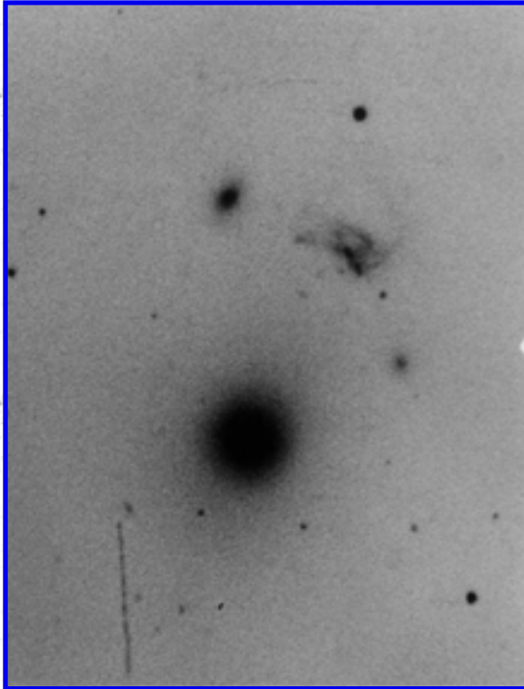
Arp 133
