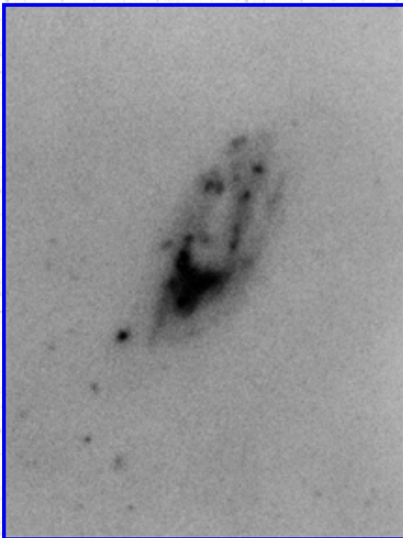
Arp 265
