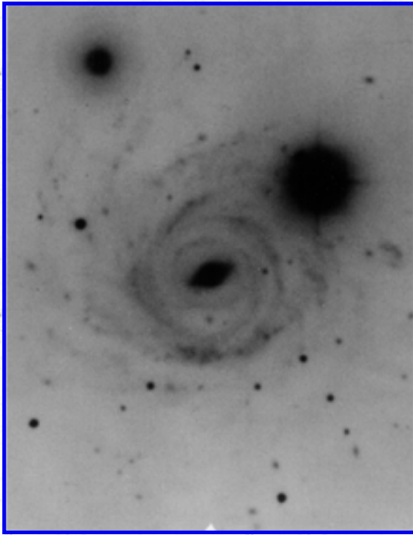
Arp 117
