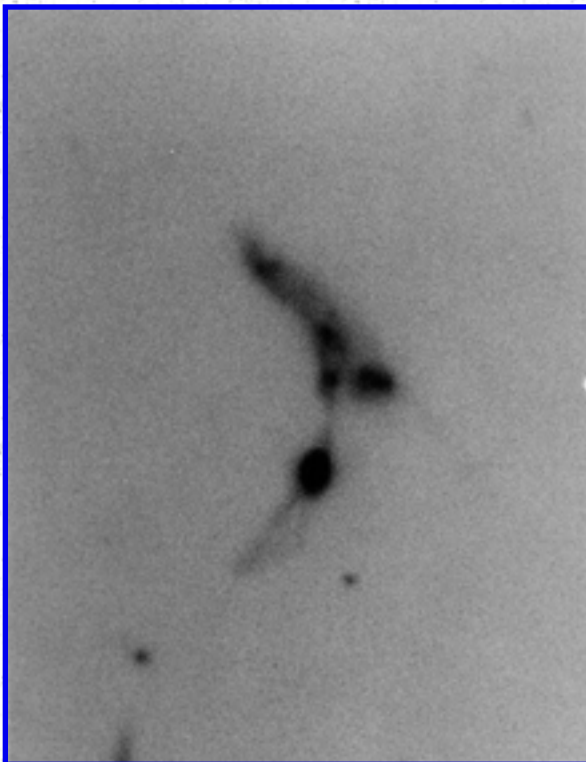
Arp 149
