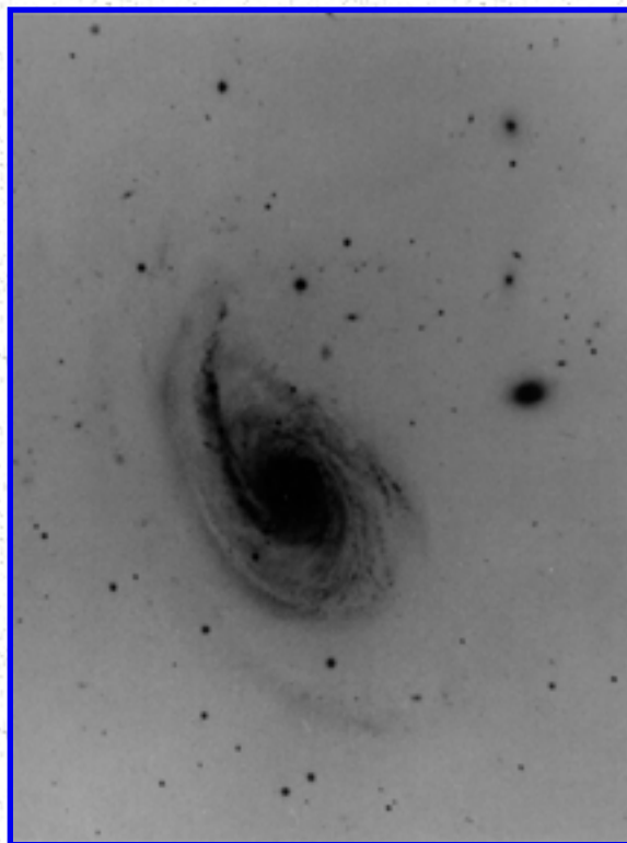
Arp 78
