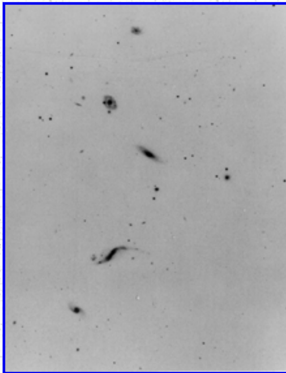
Arp 326
