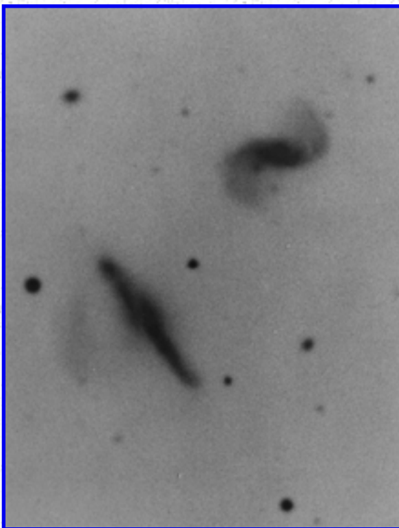
Arp 293
