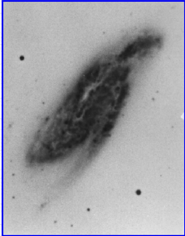
Arp 18
