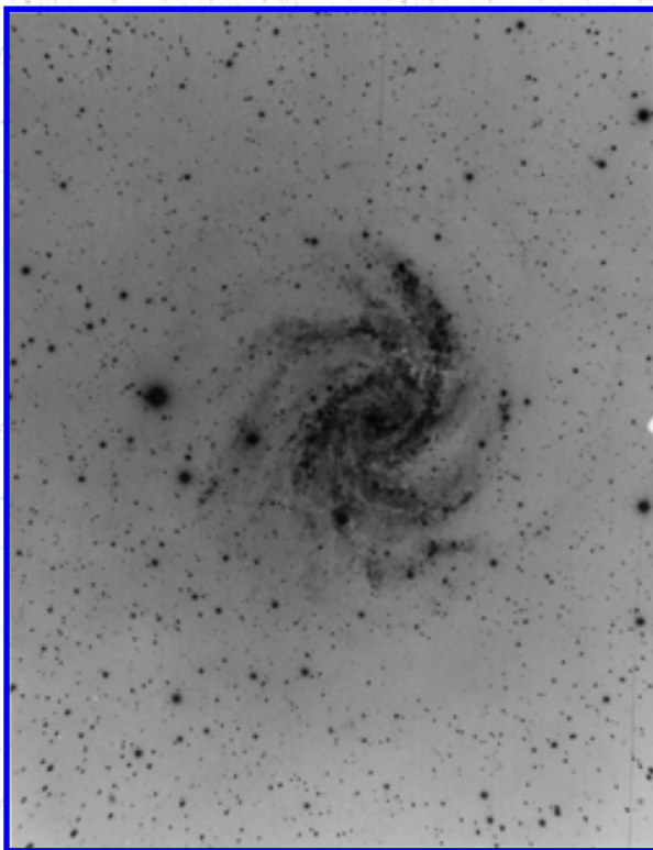
Arp 29
