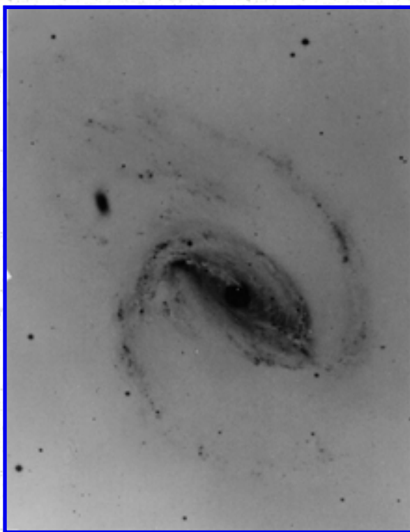
Arp 77
