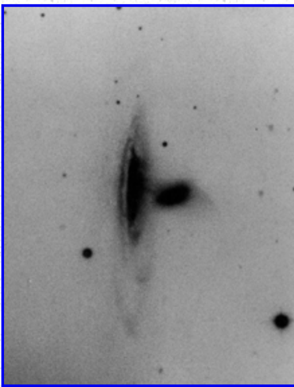
Arp 282
