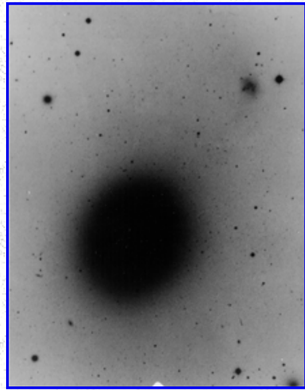
Arp 134
