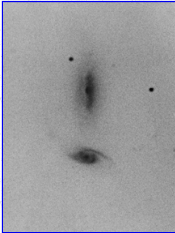
Arp 246
