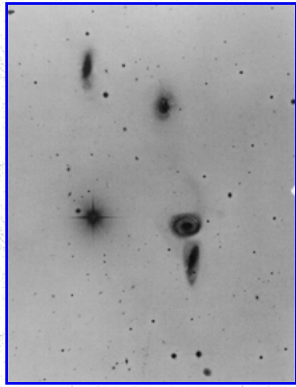
Arp 318
