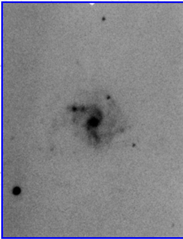
Arp 51
