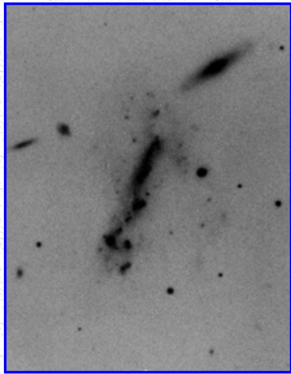
Arp 258
