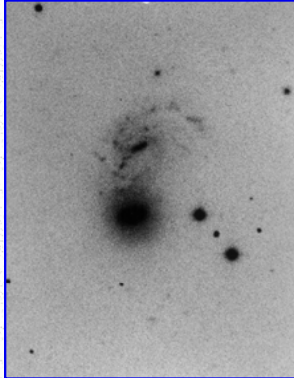
Arp 130
