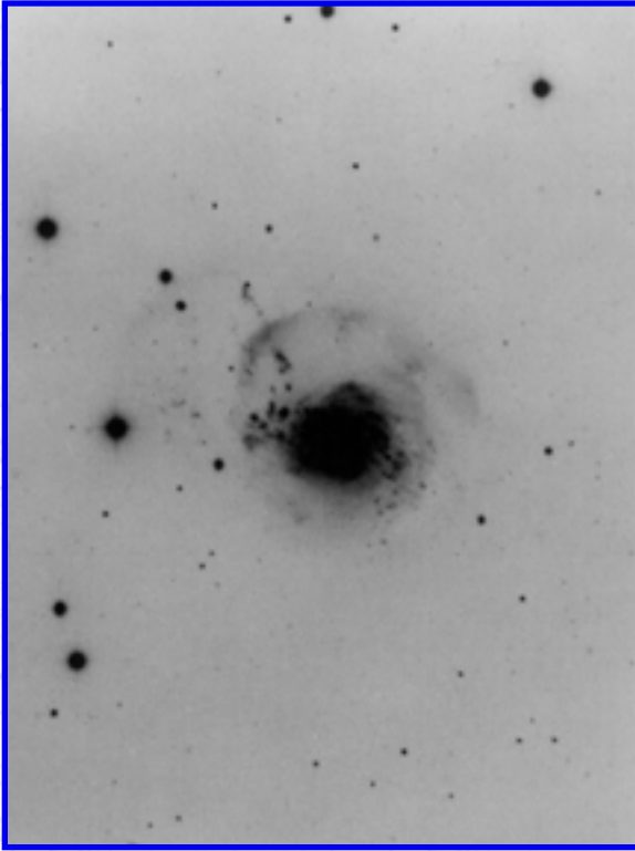
Arp 217
