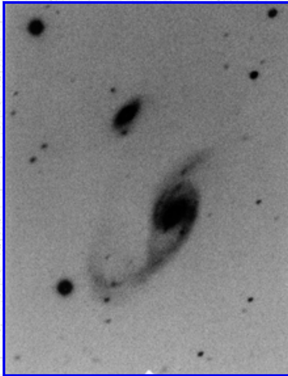
Arp 70
