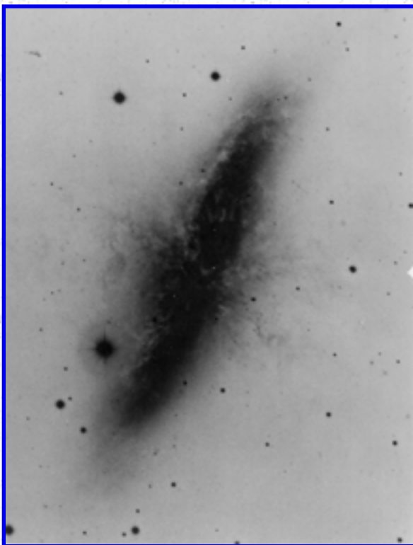
Arp 337
