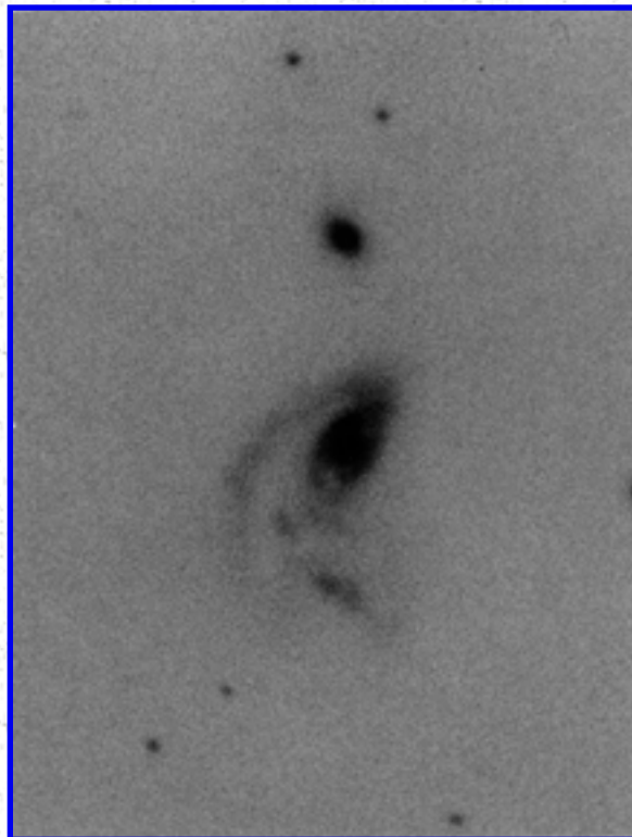
Arp 110
