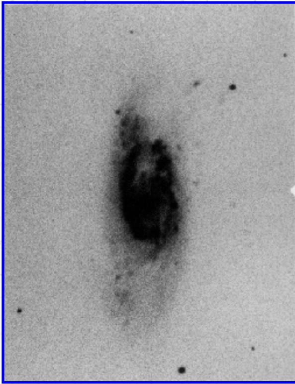
Arp 15
