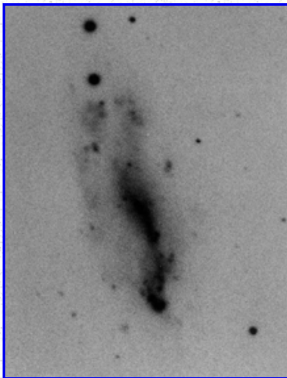
Arp 262
