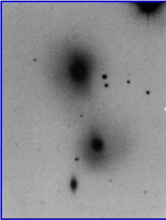
Arp 171
