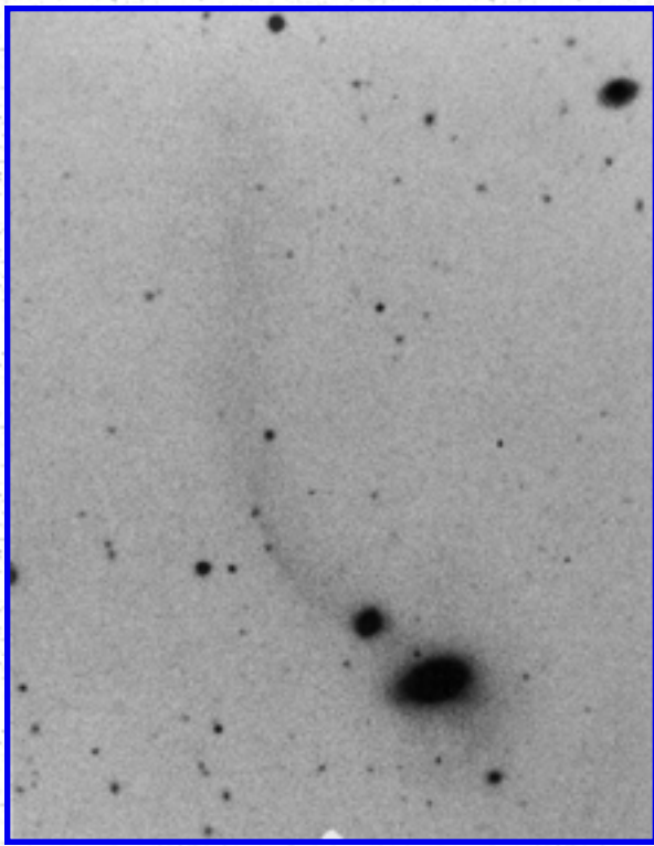
Arp 174
