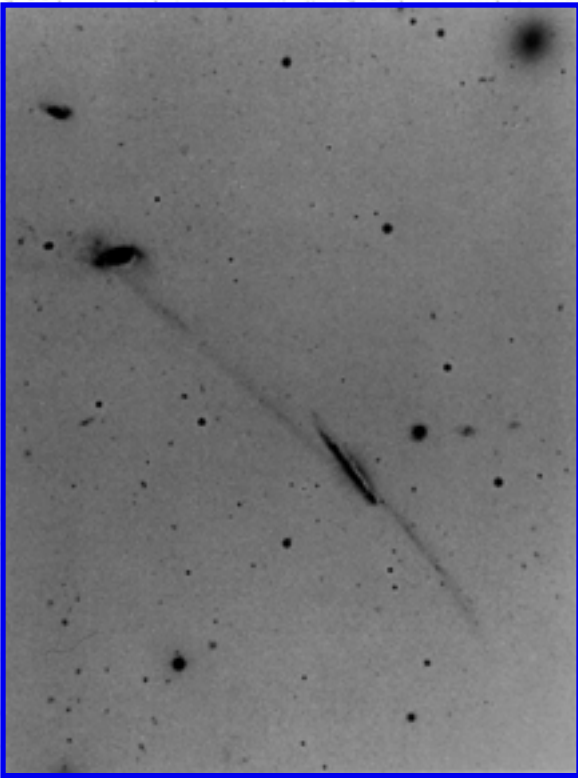
Arp 295
