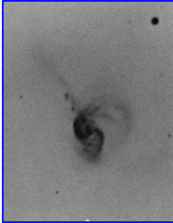
Arp 186
