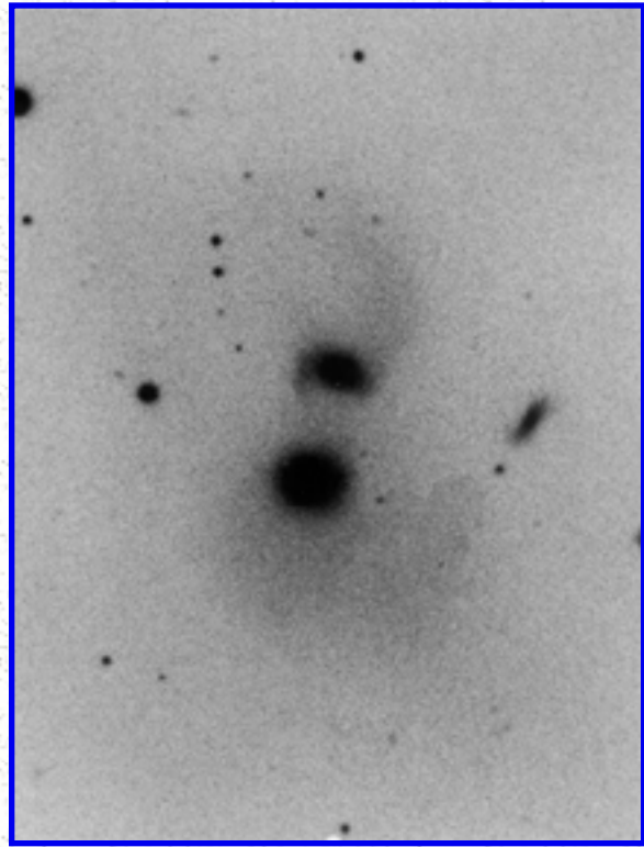
Arp 172
