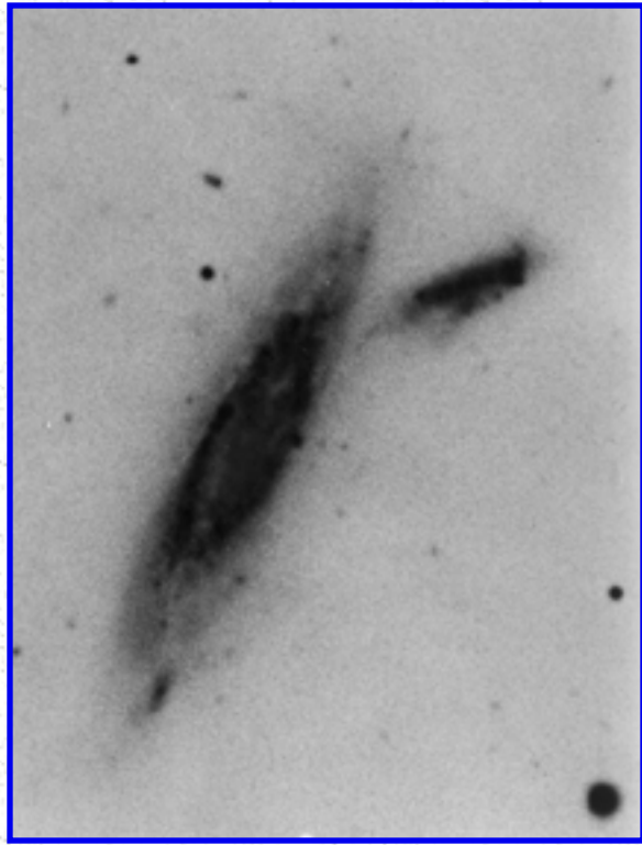
Arp 280
