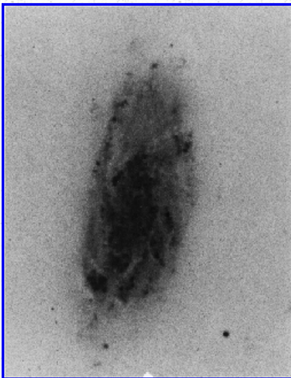
Arp 13
