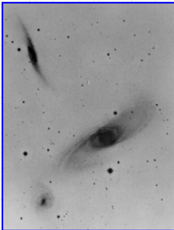
Arp 286
