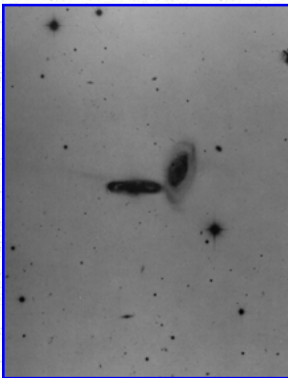
Arp 294
