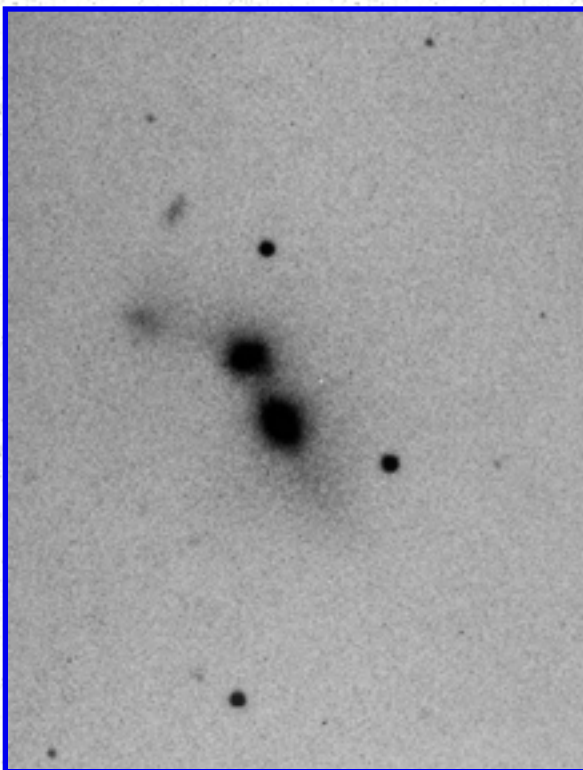
Arp 249
