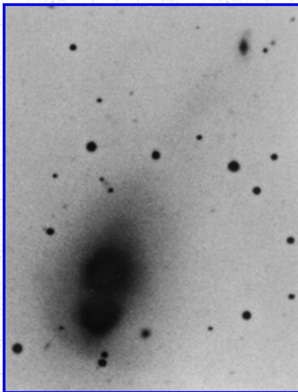
Arp 166
