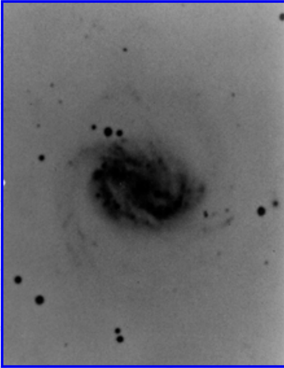
Arp 185
