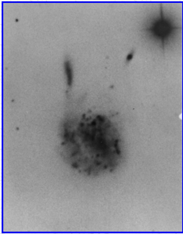
Arp 24
