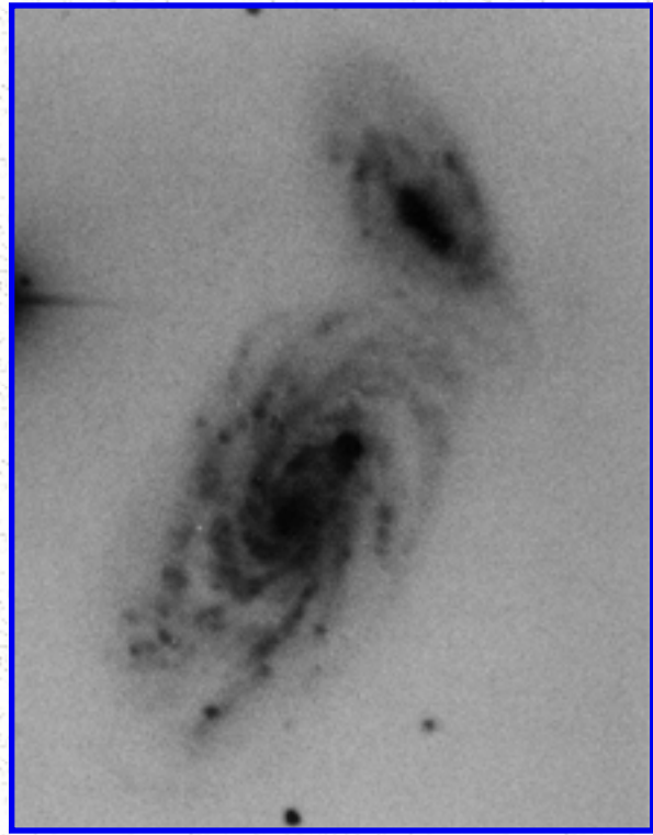
Arp 276
