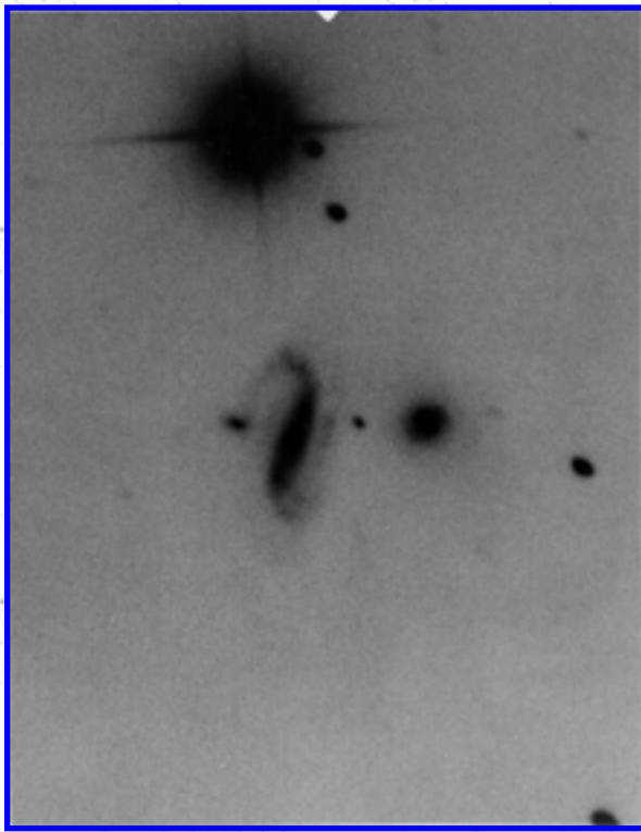
Arp 47
