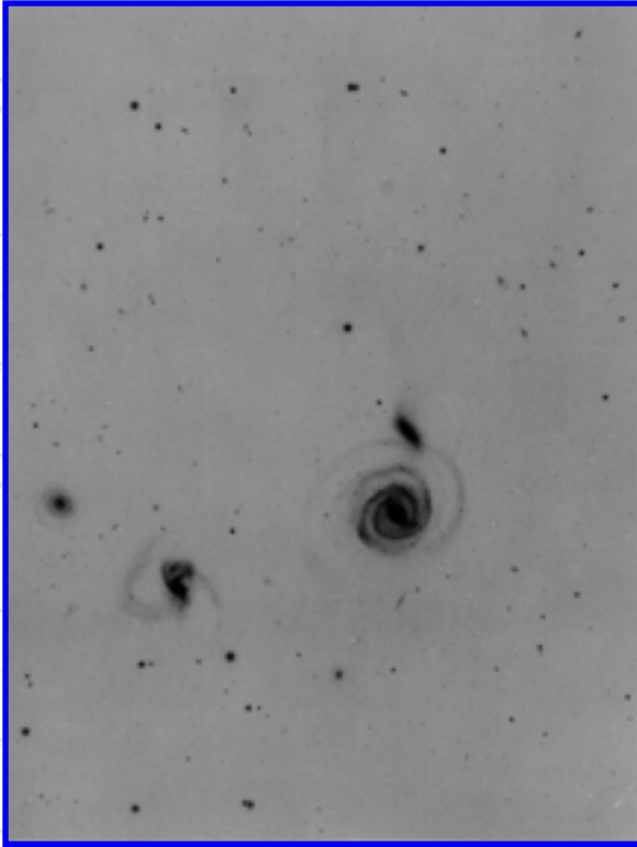
Arp 297
