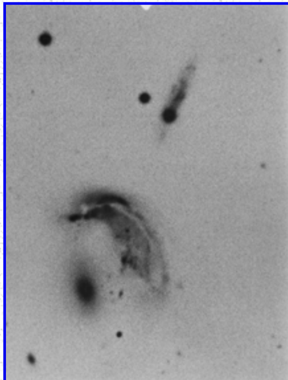
Arp 142
