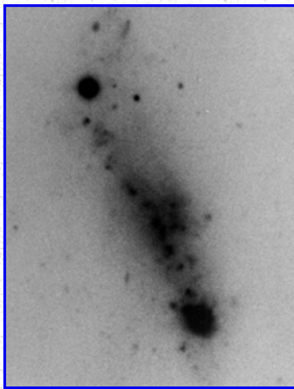
Arp 266
