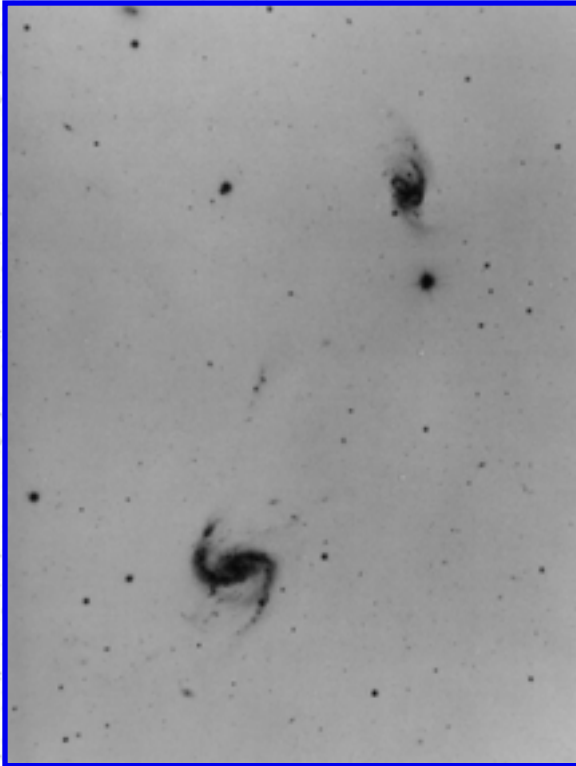
Arp 305
