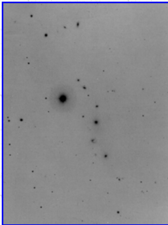
Arp 330
