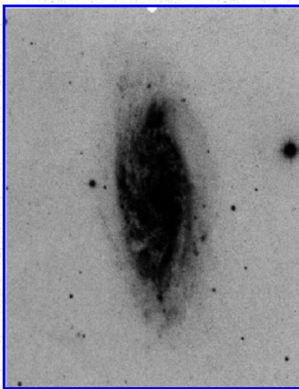
Arp 14
