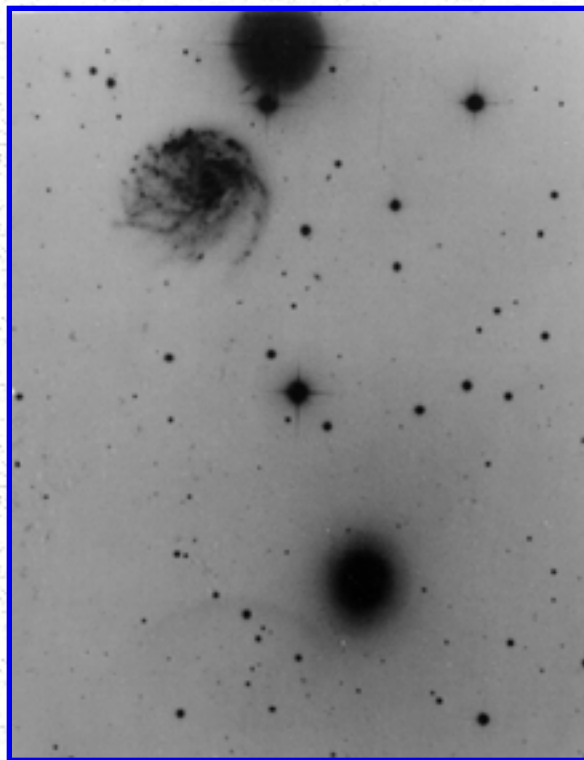
Arp 114
