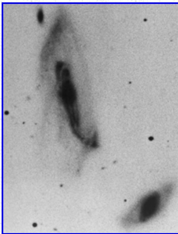
Arp 290
