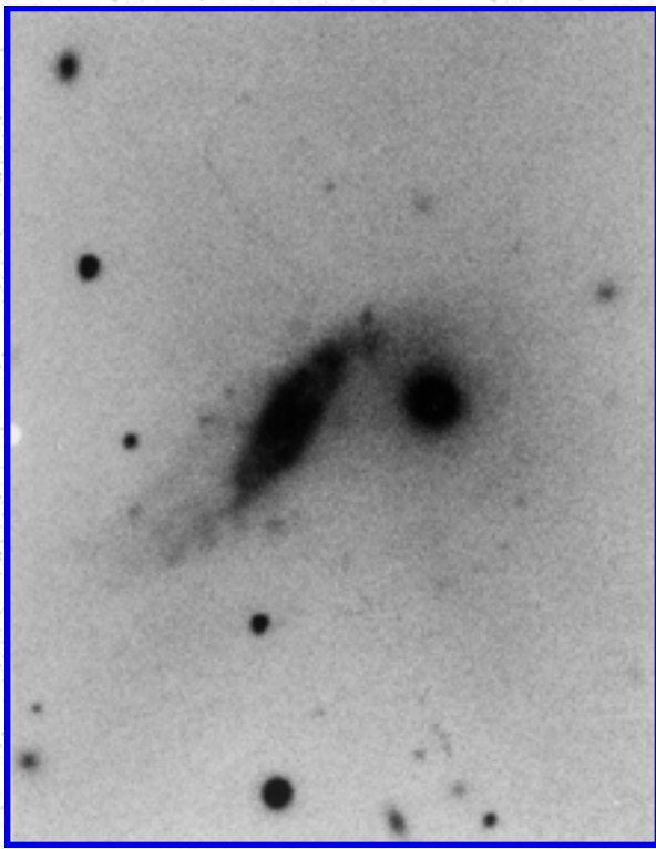
Arp 122
