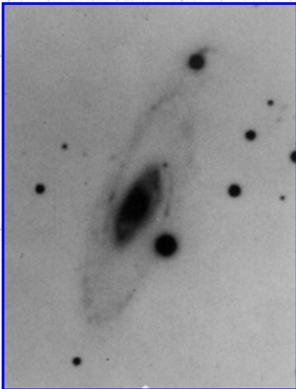
Arp 333
