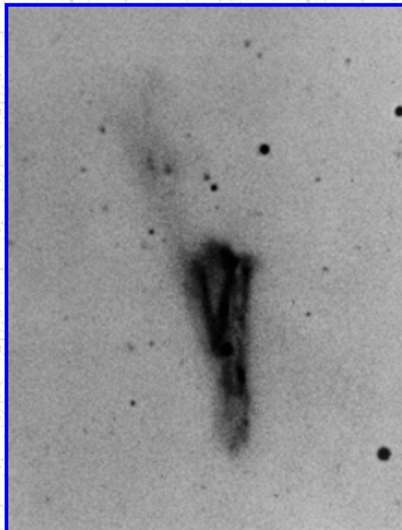
Arp 158
