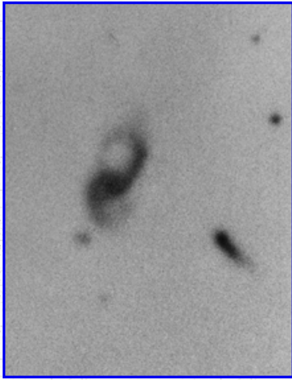
Arp 218
