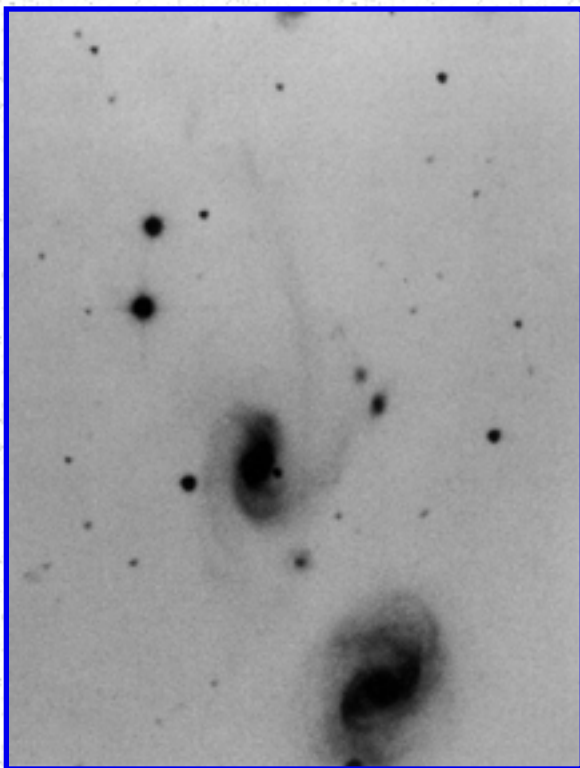
Arp 181
