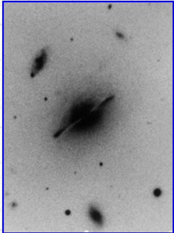
Arp 292
