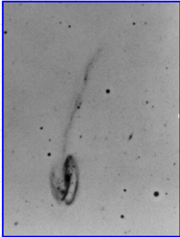
Arp 188
