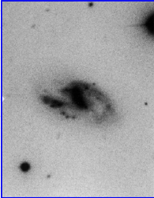
Arp 17
