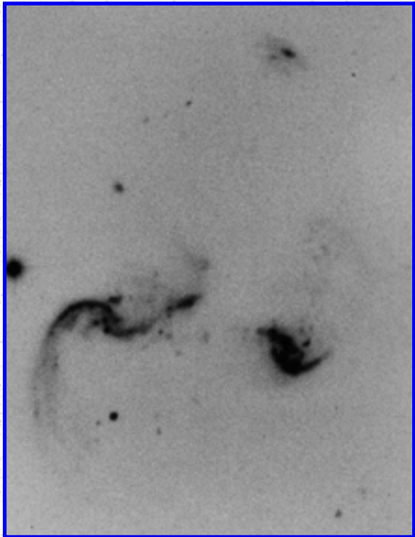
Arp 256
