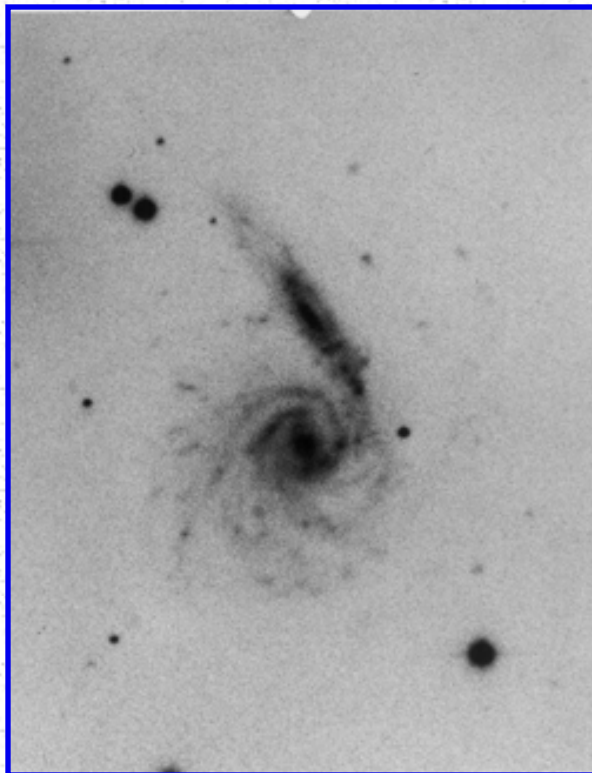
Arp 30
