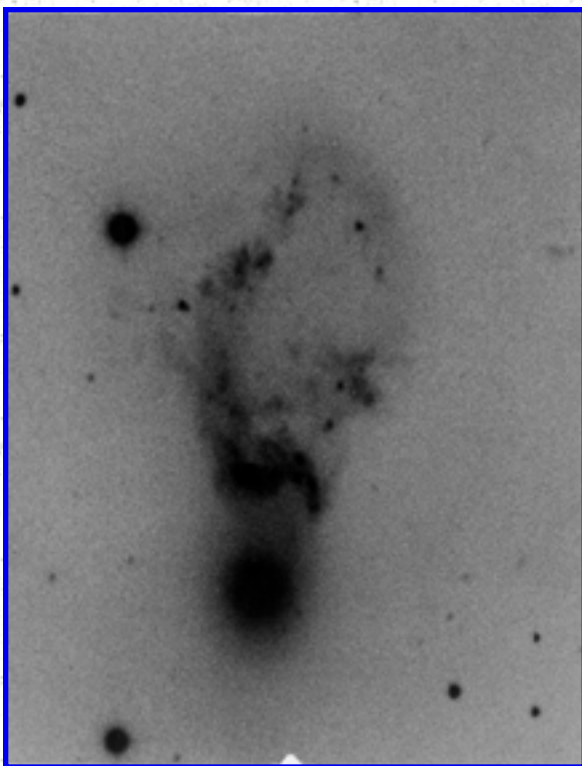
Arp 141
