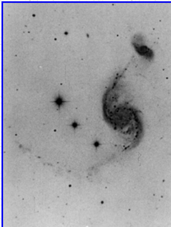
Arp 82
