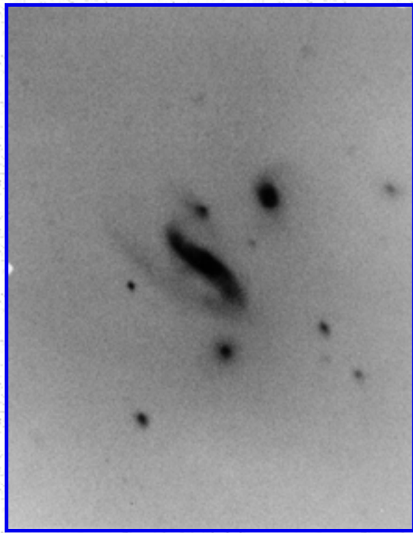
Arp 48
