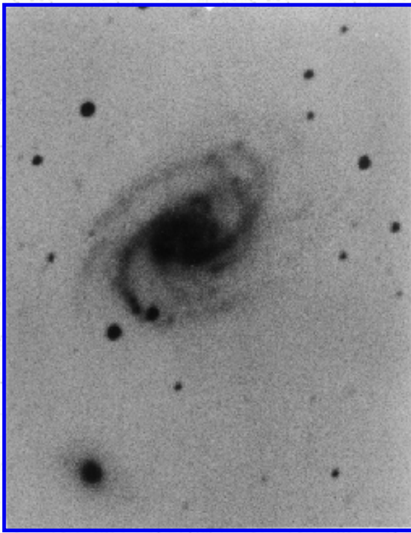
Arp 7
