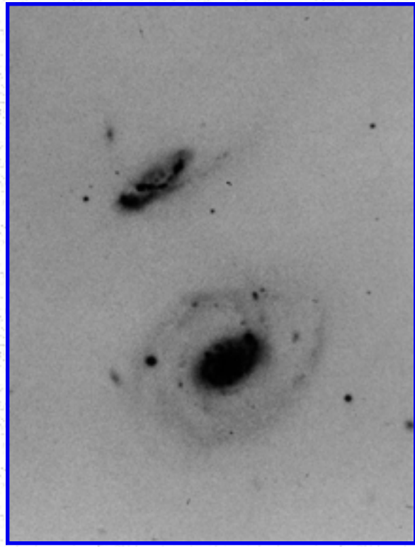
Arp 298
