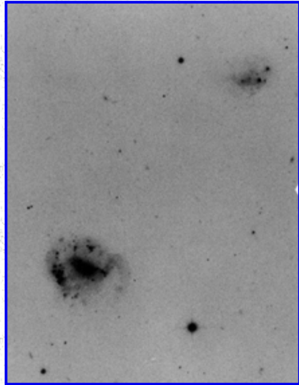
Arp 306
