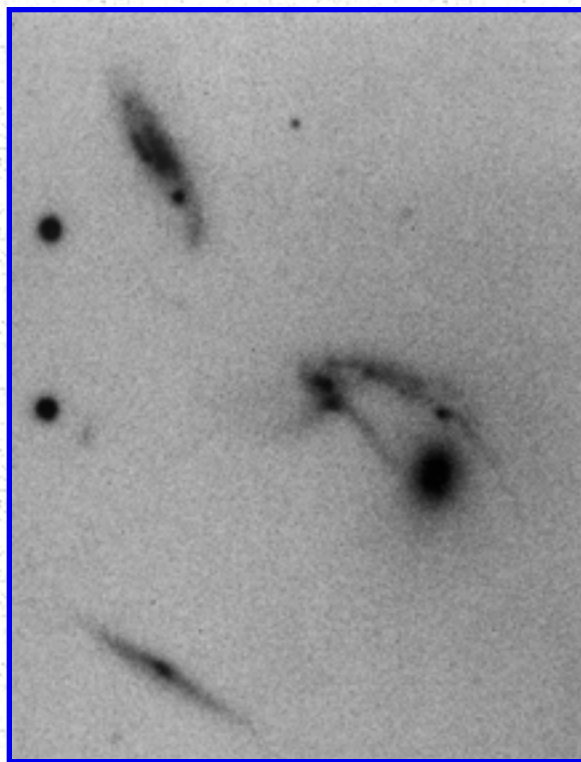
Arp 150
