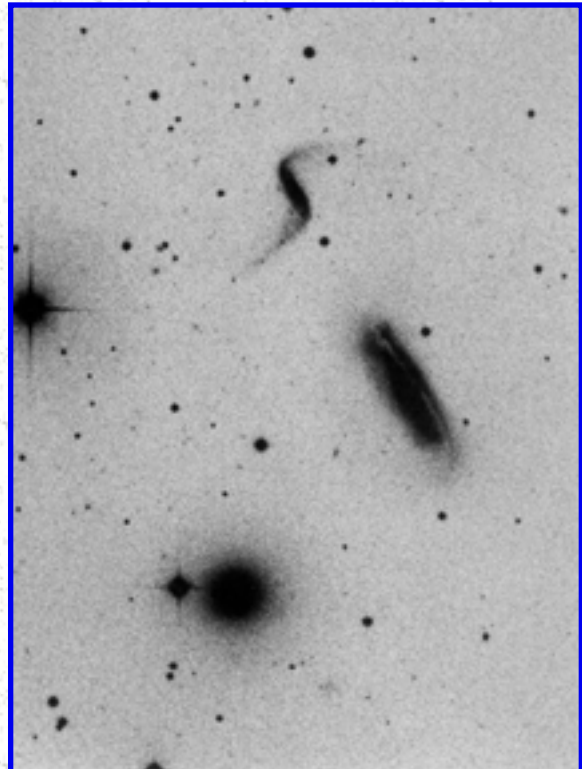
Arp 316
