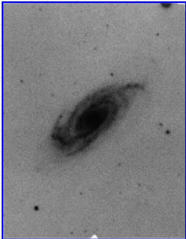
Arp 8
