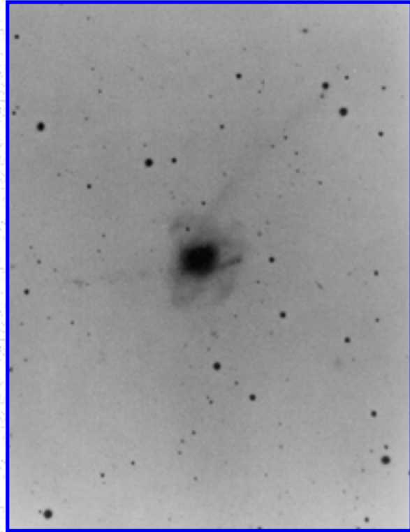
Arp 226
