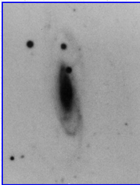
Arp 334
