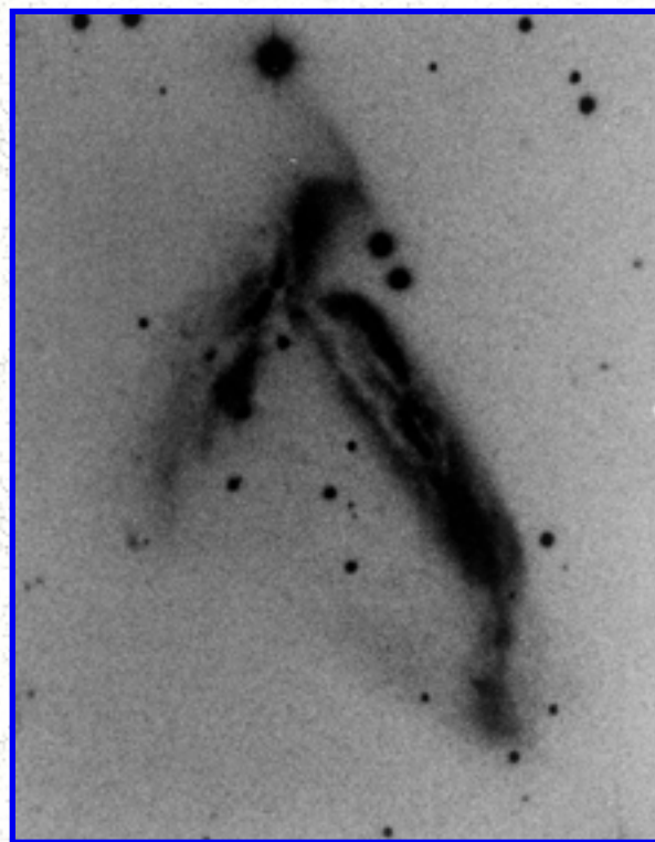
Arp 278
