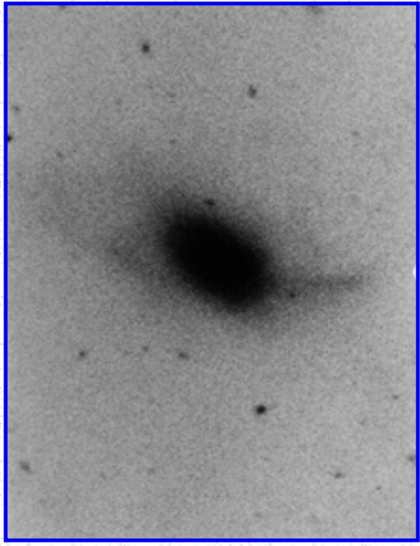
Arp 164
